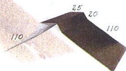
HARJALISTA
