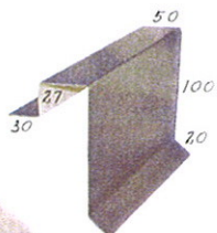
PÄÄTYLISTA
