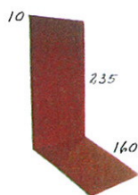
LIITOSLISTA
